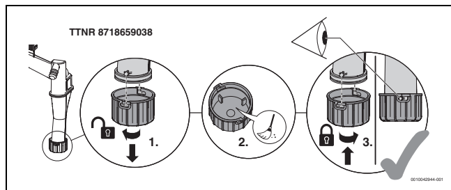
Sl.84 Čišćenje dna sifona
