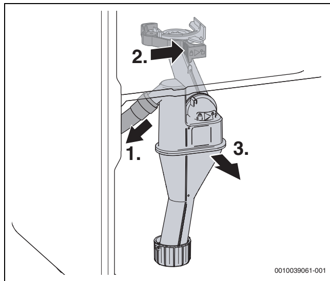
SI.83 Demontaža sifona za kondenzat
