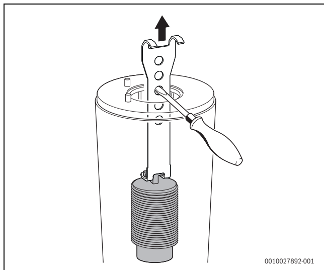
Sl.61 Vađenje donjeg elementa za raspodjelu
