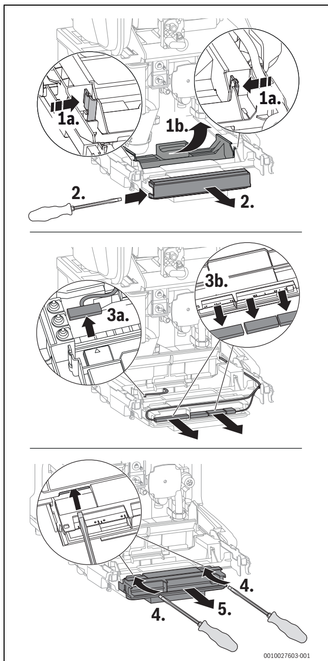
SI.82 Vađenje upravljačkog uređaja
