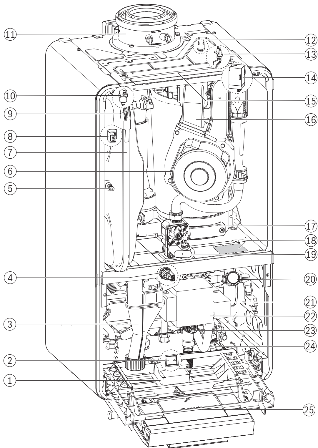
Sl.7 Pregled proizvoda - cirko uređaj
