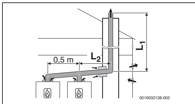
Sl. 30 Kaskada s 2 uređaja: Fiksni odvod dimnih plinova u oknu prema B 53p s dovodom zraka ovisnim o zraku u prostoriji na uređaju
