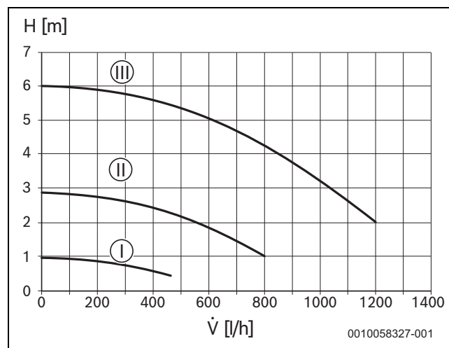
SL.45 Karakteristika Pumpa za grijanje (konstantni tlak)
