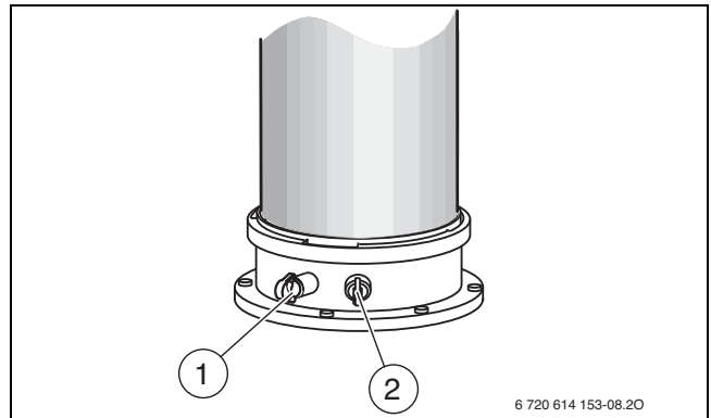
Sl. 51 Mjerni nastavak za zrak izgaranja i dimne plinove
