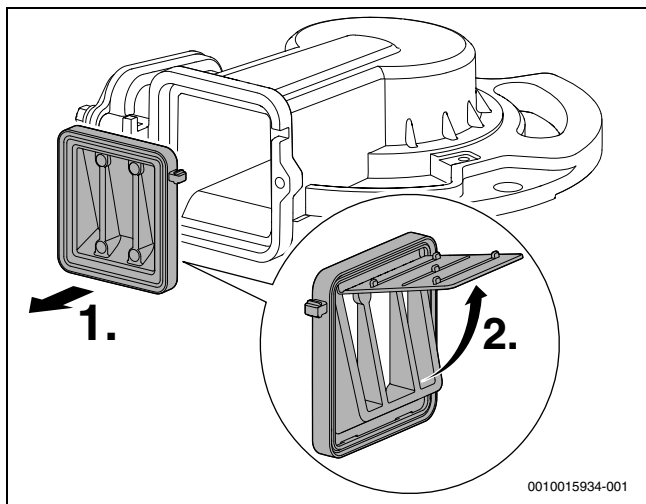
Sl.55 Provjera povratne zaklopke u uređaju za miješanje
