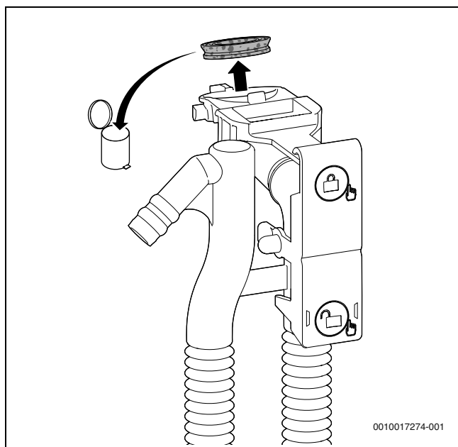
Sl. 64 Uklanjanje brtve s gornje strane sifona kondenzata
