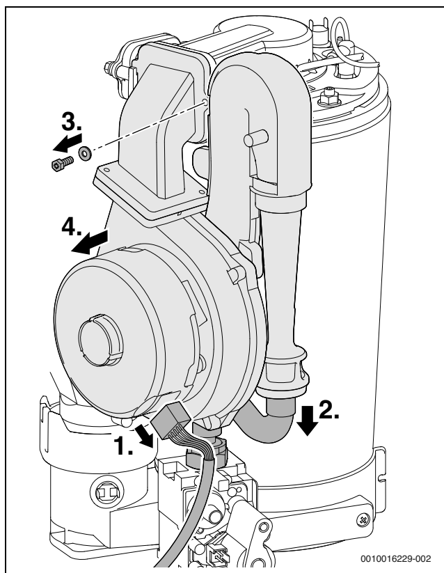
Sl.53 Demontaža ventilatora s miješalištem
