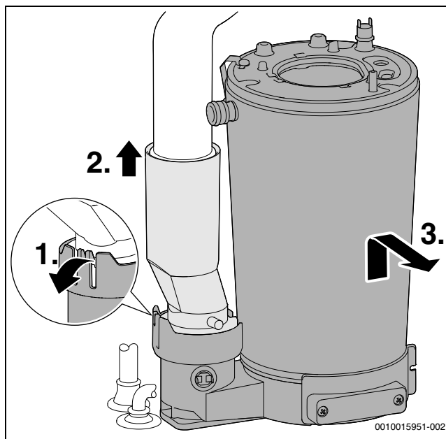
Sl.77 Demontaža toplinskog bloka
