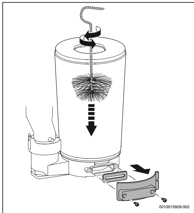
Sl.59 Očistiti toplinski blok
