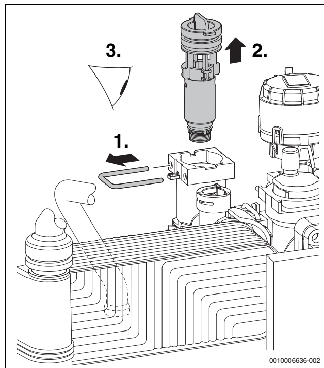
Sl. 69 Ispitivanje sita u cijevi za hladnu vodu
