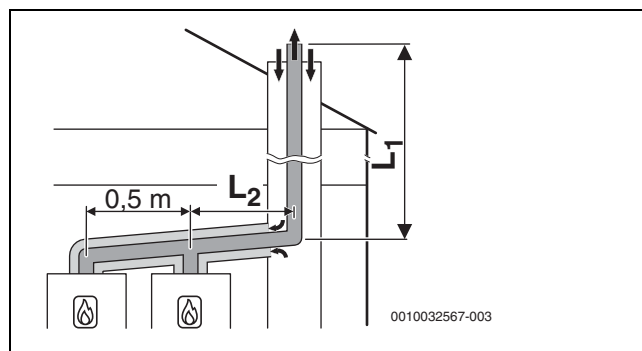
Sl. 29 Kaskade s 2 zrešaha:
