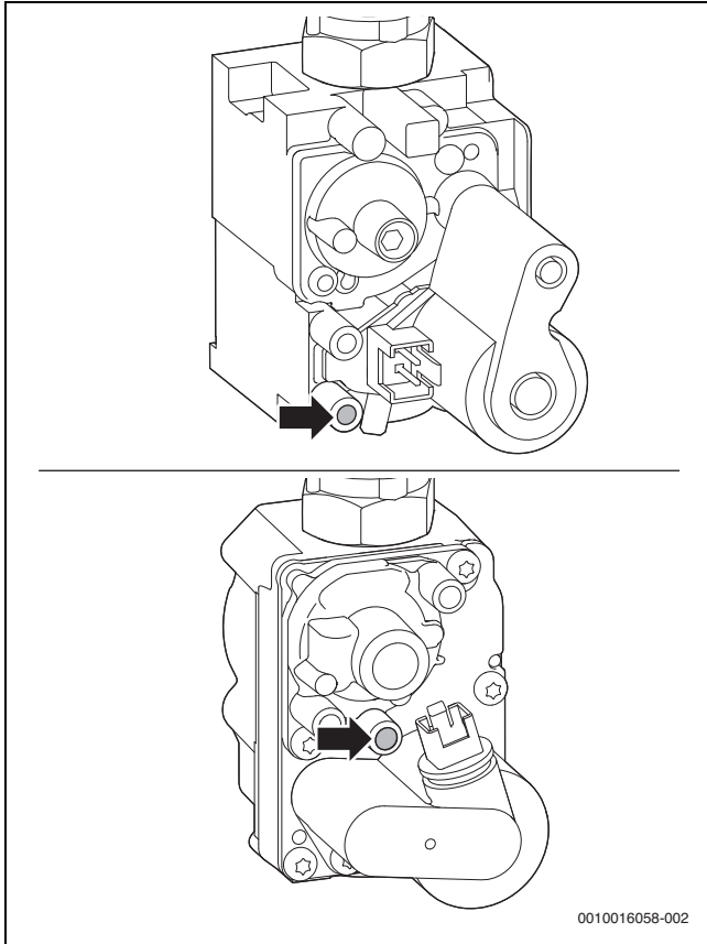
Sl. 50 Mjerni nastavci za priključni tlak plina
