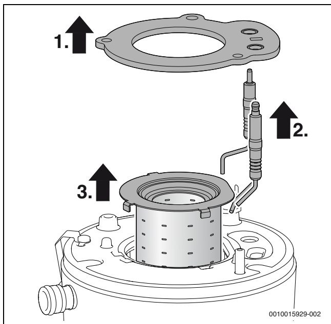
Sl.56 Skidanje plamenika
