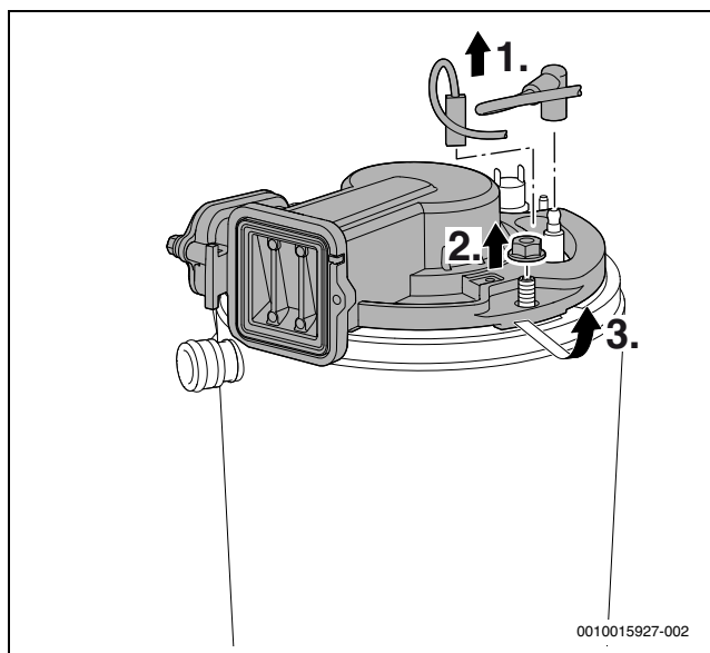
Sl.54 Otpustite poklopac plamenika
