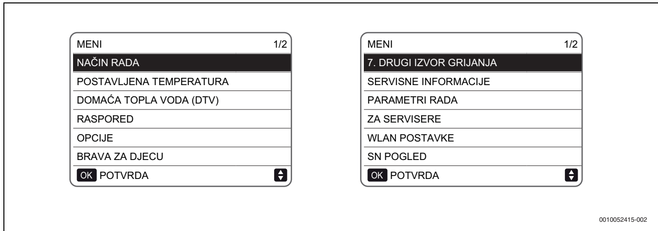
Sl.155 Izbornik
