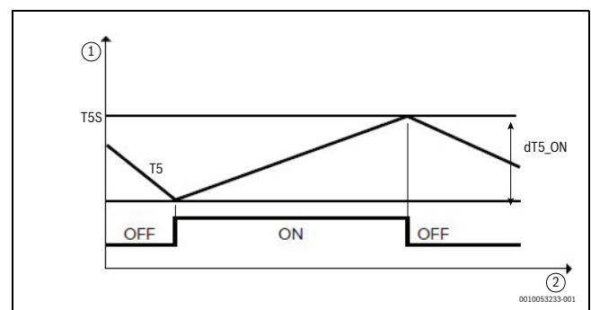
Sl.115 1.6 dt5_UKLJUČENO
