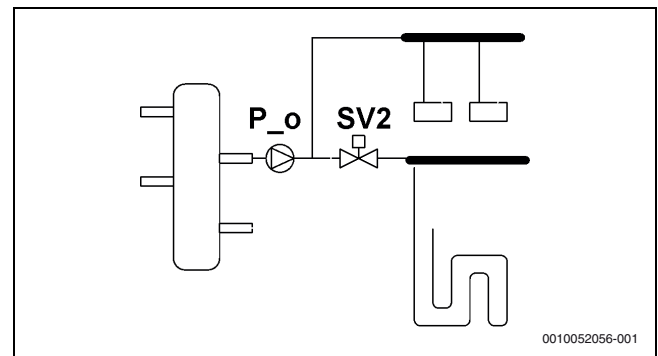
Sl.81 Dvozonska instalacija
