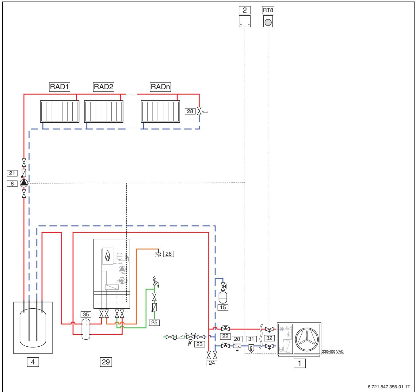
Sl.26 Vanjska jedinica s jednim ili više krugova grijanja i vanjskim pomoćnim grijačem (CS2000AWF 4-6 R-S, CS2000AWF 8-10 R-S, CS2000AWF 12-16 R-S/T)
