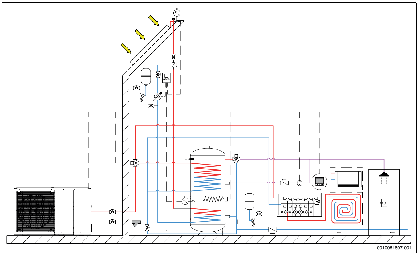
Sl.52 Vodeni priključci
