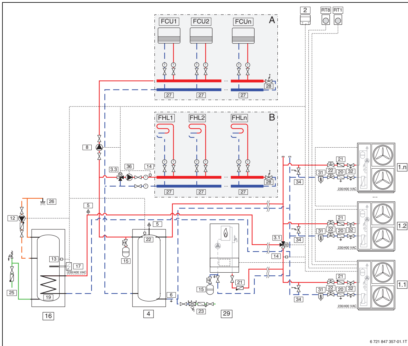
Sl.27 Vanjska jedinica s jednim ili više krugova grijanja, vanjskim dodatnim grijačem, spremnikom sanitarne tople vode i kaskadnim (CS2000AWF 18-30 R-T)
