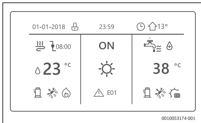
Sl. 152 Zaslona
