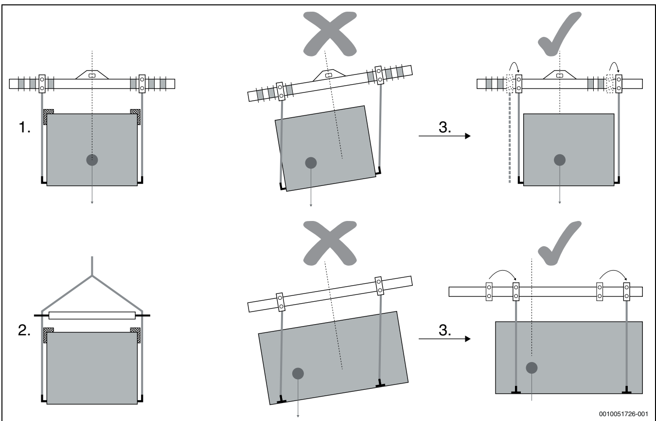
Sl.29 Podizanje
