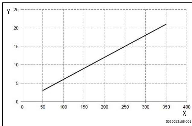
Sl.56 Ukupna zapremina ekspanzijske posude (veličine CS2000AWF 4 R-S do CS2000AWF 16 R-S/CS2000AWF 16 R-T)
