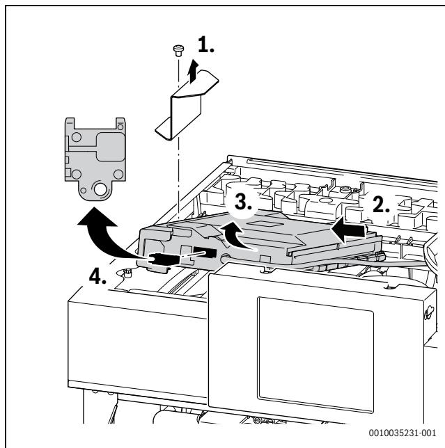
Sl.49 Zamjena kodnog utikača
