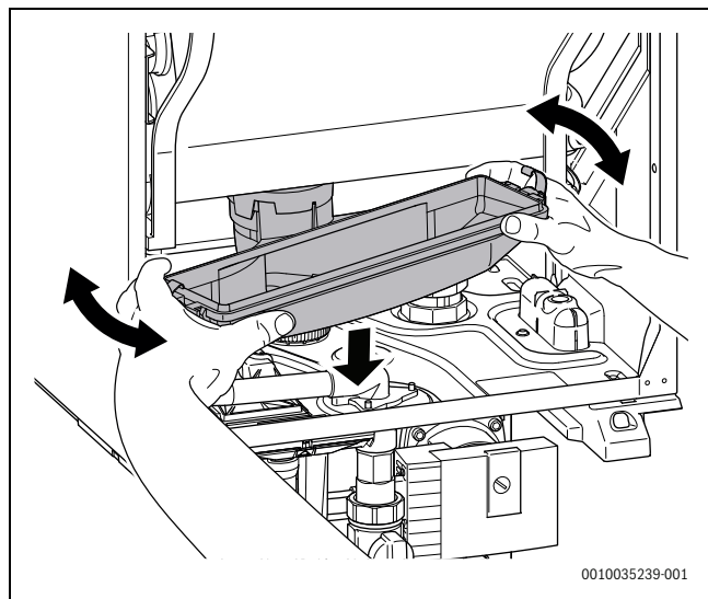
Sl. 46 Uklonite posudu za skupljanje kondenzata.
