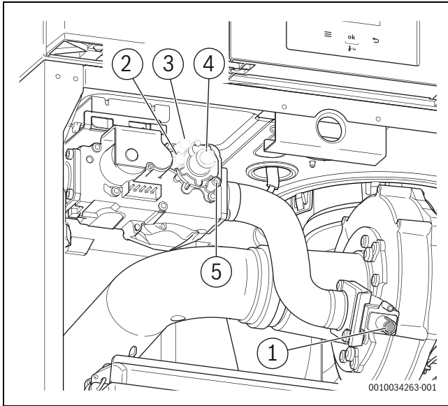
Sl.33 Pregled priključaka za ispitivanje i podesnih vijaka \geq 85 kW
