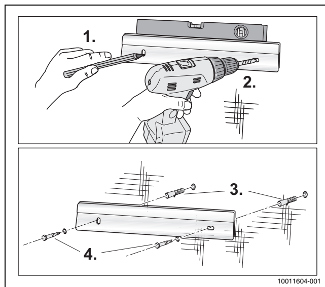
Sl.11 Montaža nosača na betonski zid
