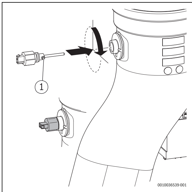
Sl.48 Zamjena temperaturnog osjetnika dimnih plinova
