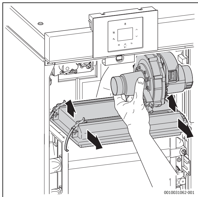
Sl.40 Demontirajte jedinicu plin/zrak zajedno s poklopcem plamenika.
