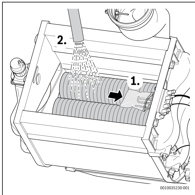
Sl.43 Čišćenje izmjenjivača topline
