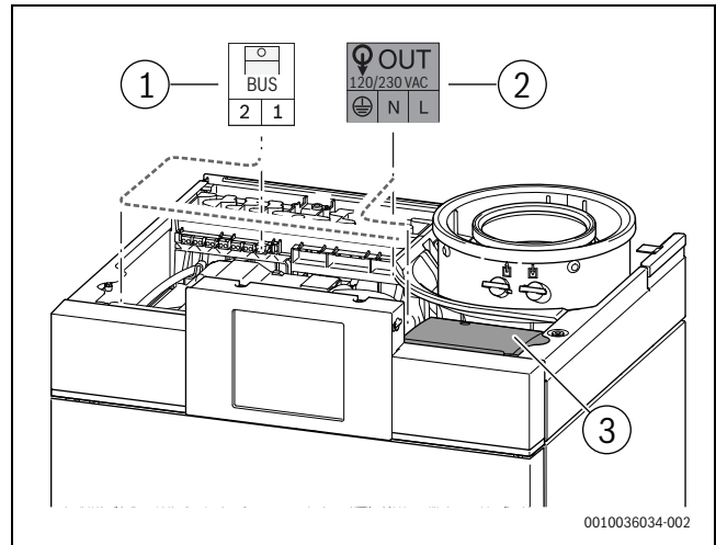
Sl.30 Montaža funkcijskog modula
