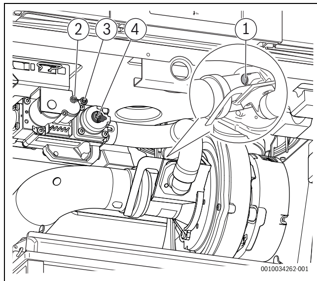
Sl.32 Pregled priključaka za ispitivanje i podesnih vijaka ≤ 70 kW
