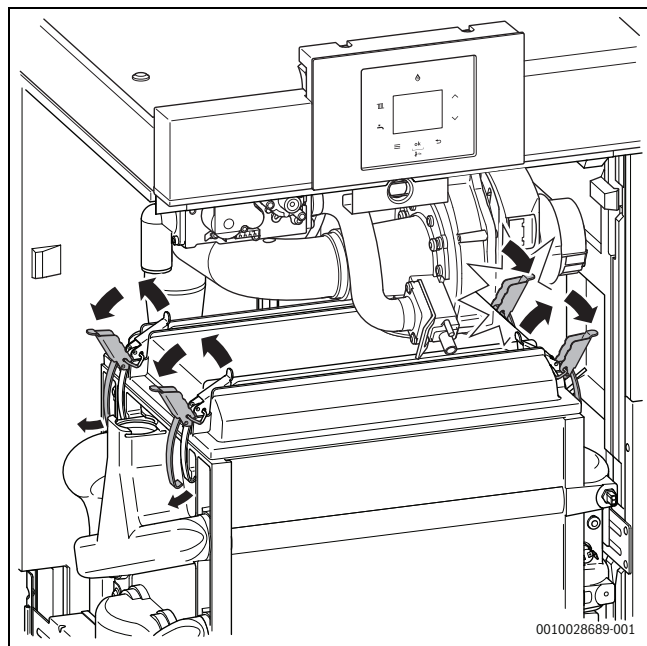
Sl.39 Otvaranje zatvarača
