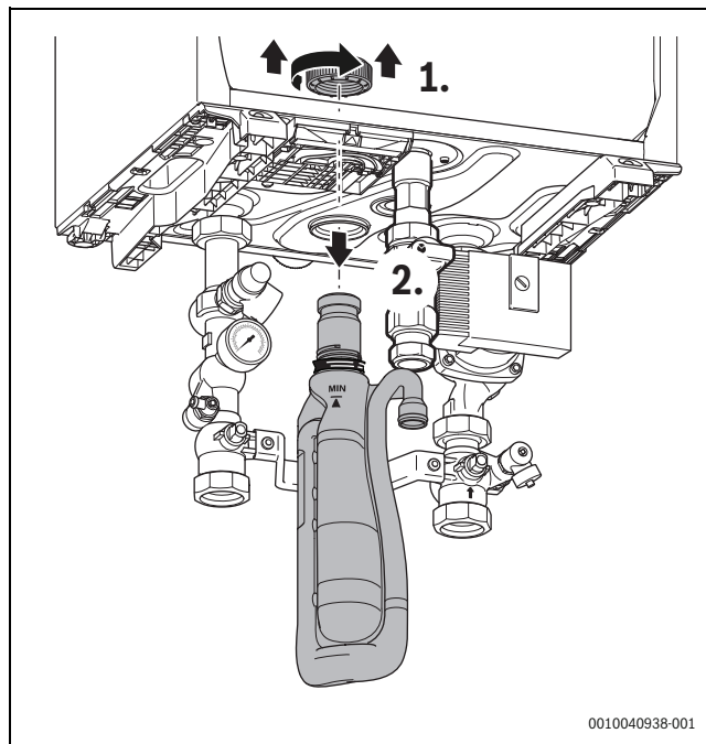
Sl.44 Demontaža sifona kotla(uređaja)
