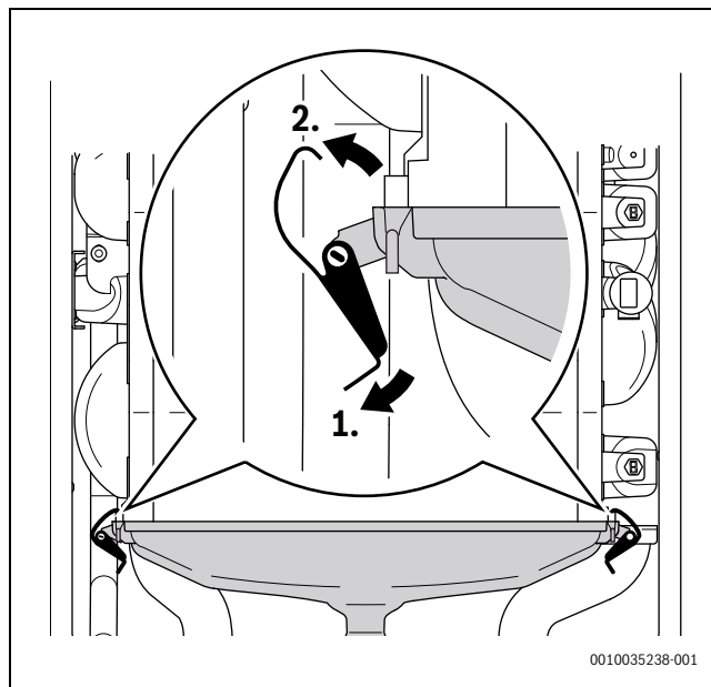
Sl.45 Otvaranje zatvarača na posudi za skupljanje kondenzata
