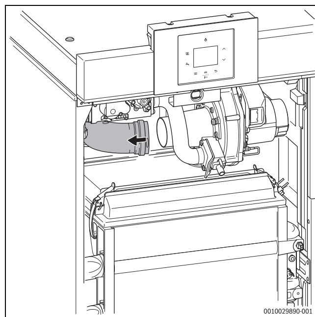
Sl.38 Demontaža usisne cijevi za zrak
