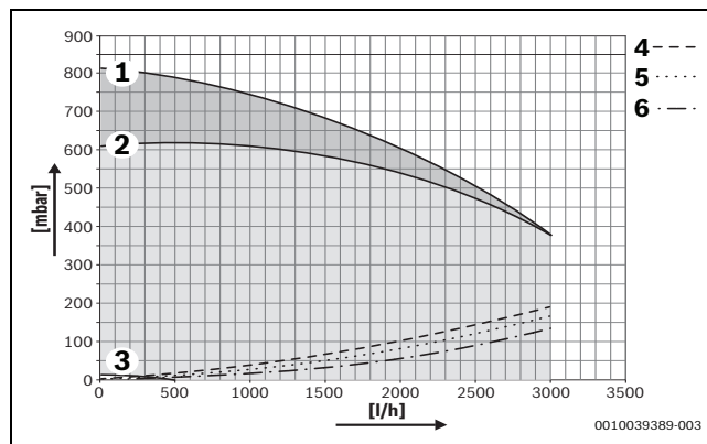
SL.51 Preostala visina isporuke pumpe 50kW-85kW
