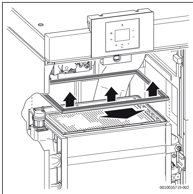
Sl.41 Uklanjanje brtve plamenika
