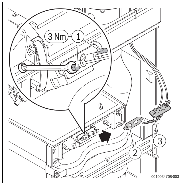
SI.47 Umetanje elektrode
