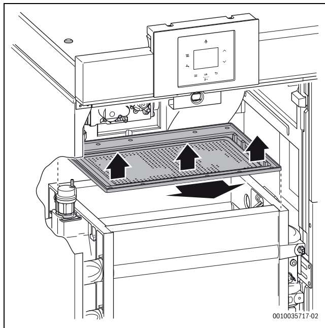
Sl.42 Uklanjanje plamenika
