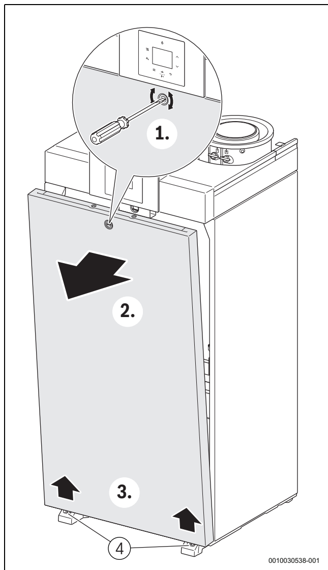
Sl.6 Otvoranje prednjeg poklopca
