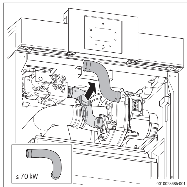
Sl.37 Demontaža crijeva za plin ≥ 85 kW
