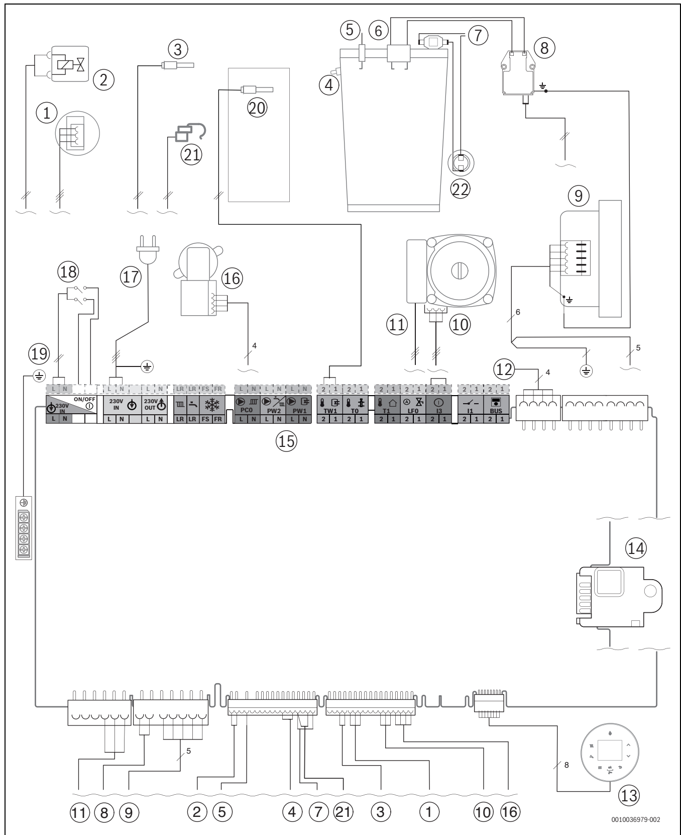
Sl.90 Električno ožičenje
