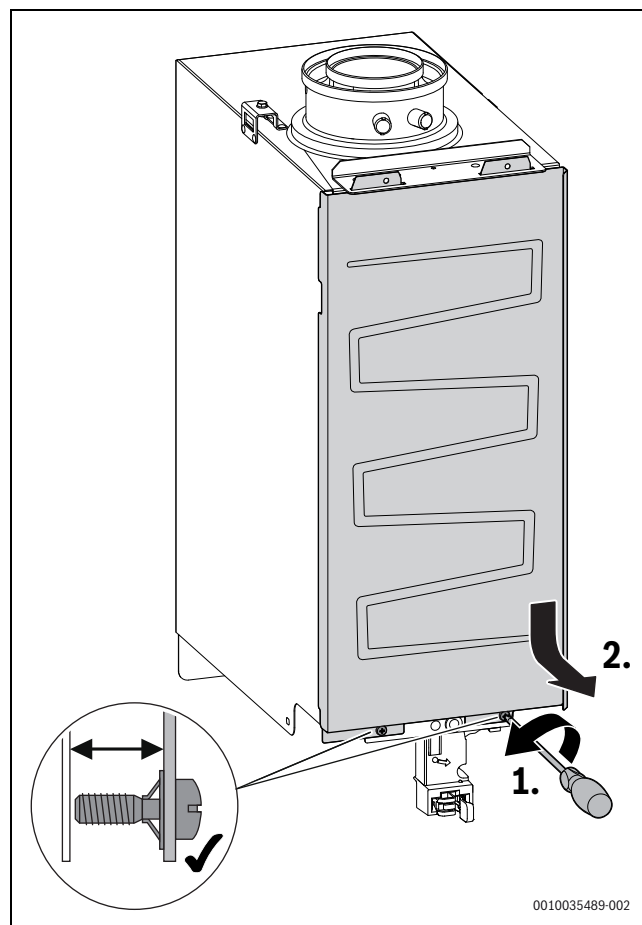
SI.50 Skidanje poklopca plamenika
