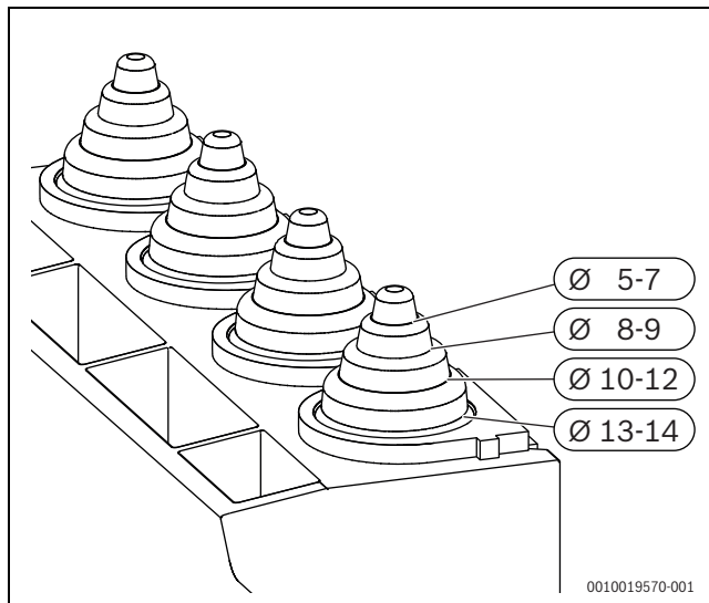
Sl.45 Prilagodba pričvrsnice kabla na promjer kabla
