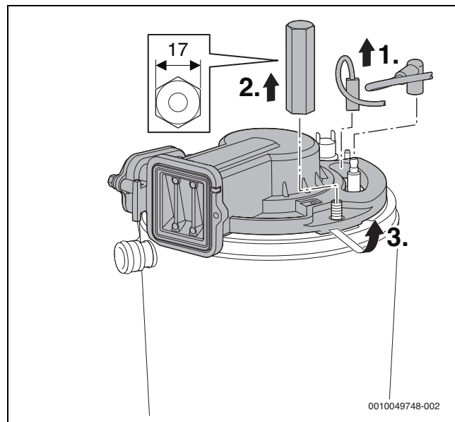
SI.59 Otpustite poklopac plamenika
