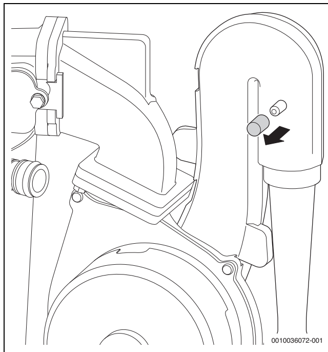
Sl. 56 Mjesto za mjerenje na uređaju za miješanje
