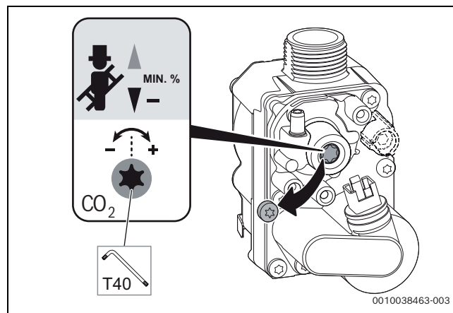
SI.54 Postavljanje udjela \text{CO}_2/\text{O}_2 pri minimalnoj nazivnoj toplinskoj snazi
