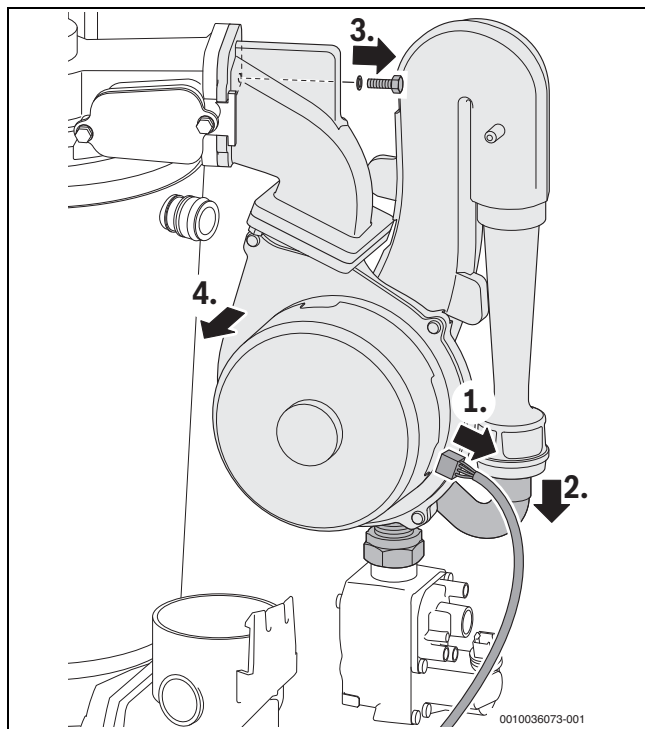
SI.58 Demontaža ventilatora s miješalištem
