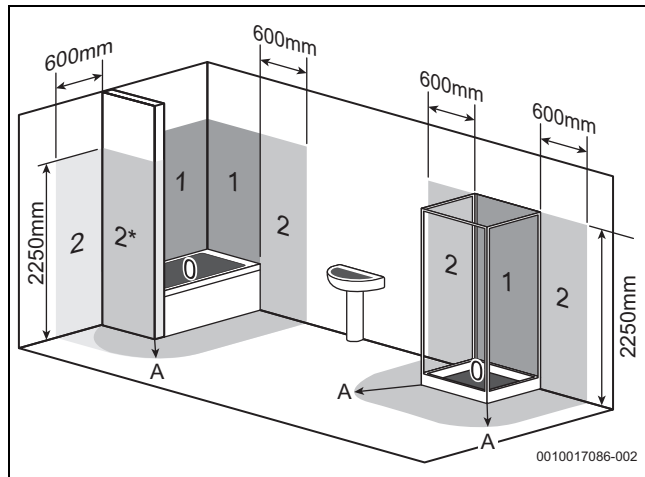
Sl.28 Zaštitna područja (primjer)
