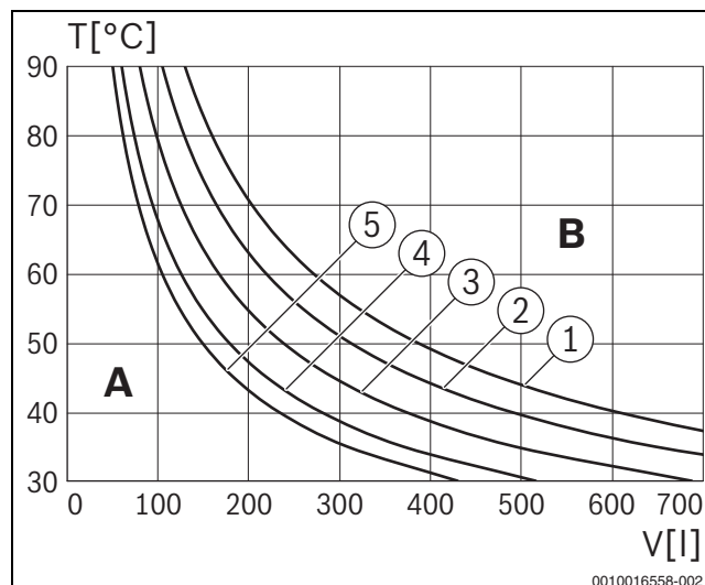
Sl.31 Karakteristike ekspanzijske posude
