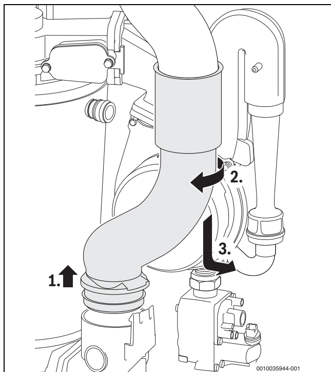
SI.57 Demontaža dimovodne cijevi
