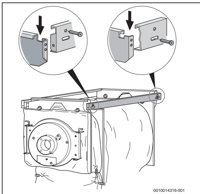
Sl.17 Zakačiti bočne traverze te ih vijčano pričvrstiti
