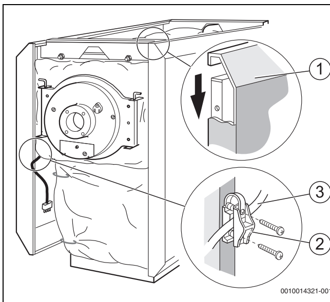
Sl.19 Zakačiti bočne stijenke i priključiti kabel plamenika
