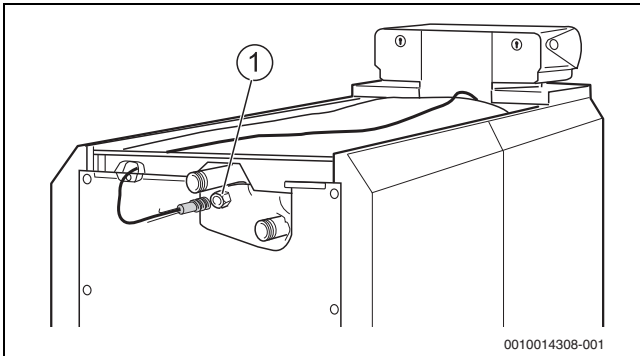
Sl.25 Uvođenje temperaturnog osjetnika u uronsku čahuru
