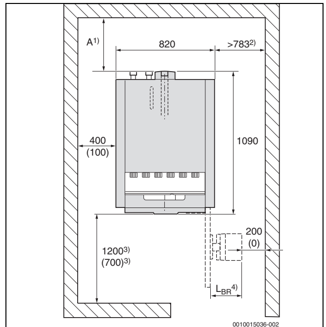
Sl.7 Prostor za postavljanje, mjere u mm → tabl. 10, str. 15 (vrijednosti u zagradama minimalni su razmaci)
