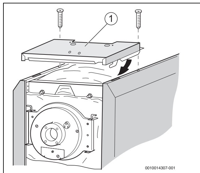
Sl.21 Montaža prednjeg poklopca kotla
