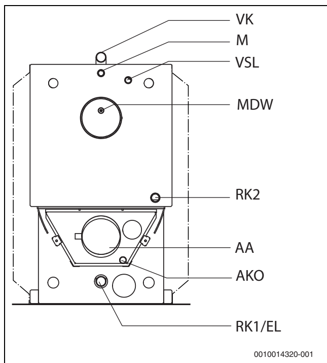
Sl.12 Priključci kotla
