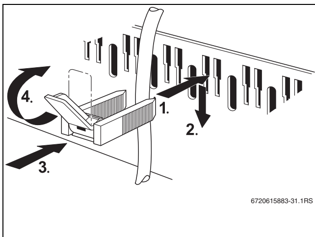
Sl.32 Kabel osigurati kabelskom objumicom
