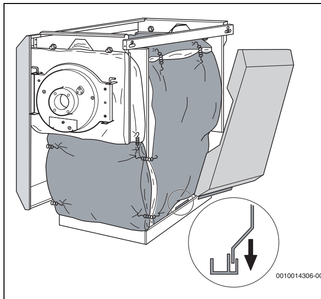
Sl.18 Umetnuti bočne stijenke
