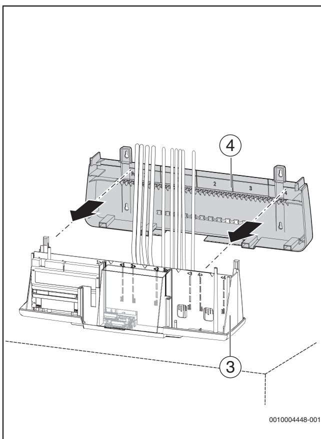
Sl.33 Montaža na kotlu, postavljanje i uglavljivanje stražnje stijenke
