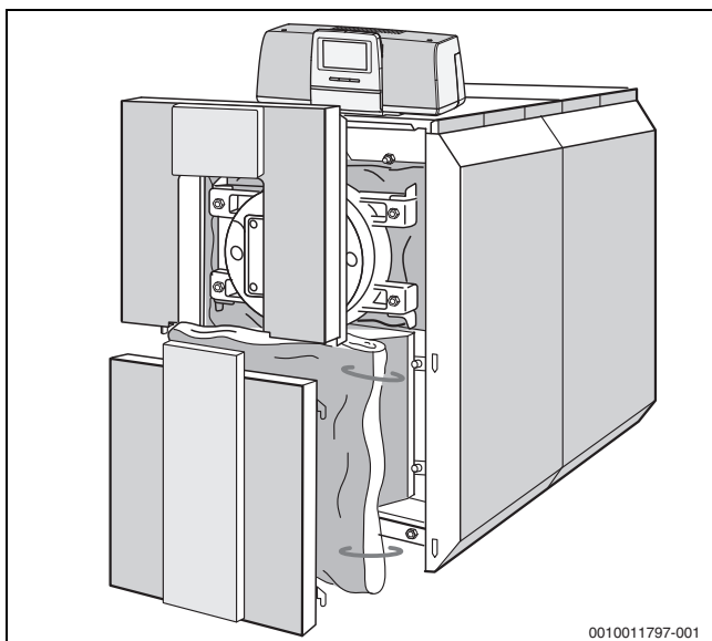
Sl.39 Skinuti prednju stijenku i prednju toplinsku izolaciju
