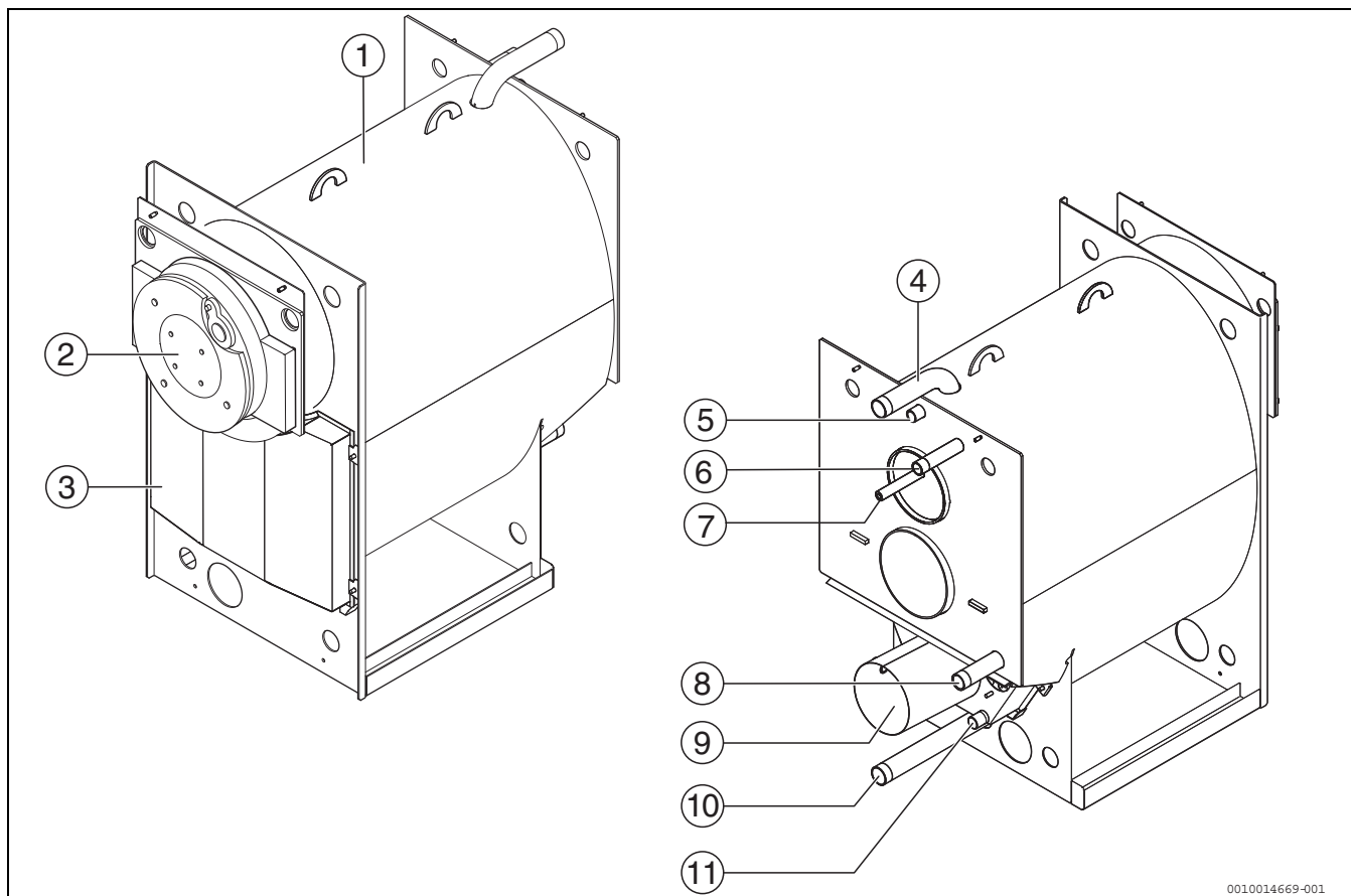
SI.2 Pregled kotla
