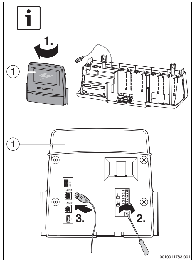
Sl.36 Podešavanje adrese regulacijskog uređaja
