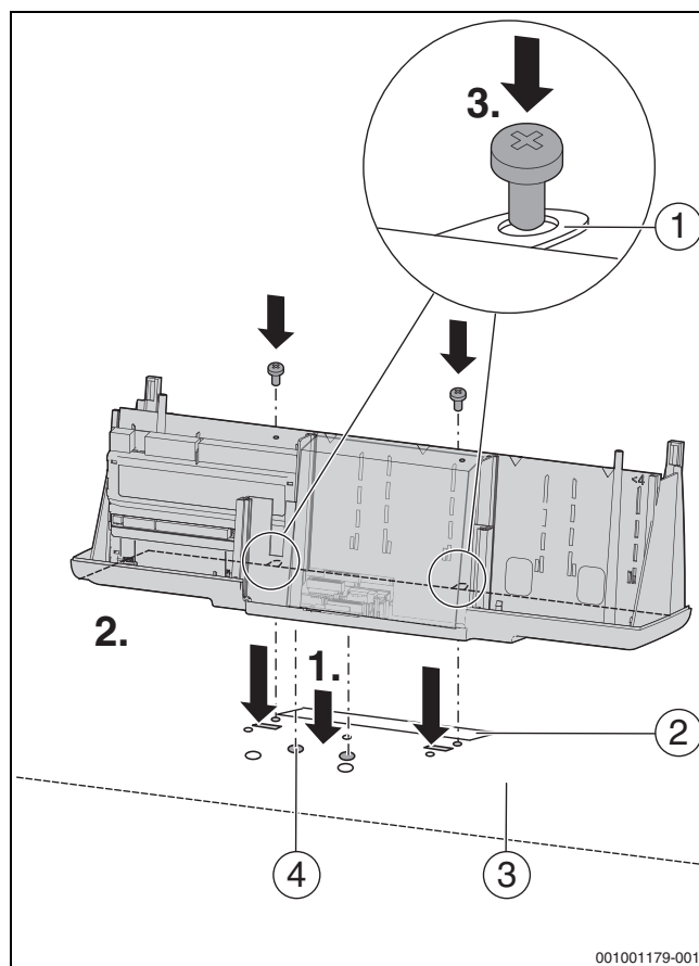
Sl.31 Montaža regulacijskog uređaja
