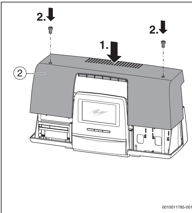
Sl.38 Montaža poklopca na regulacijski uređaj
