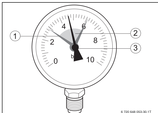
Sl. 43 Manometar za zatvorene instalacije grijanja
