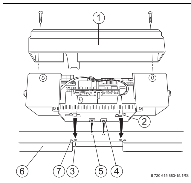
Sl.27 Montaža regulacijskog uređaja
