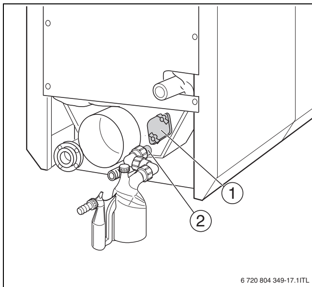
Sl.42 Poklopac za čišćenje na kolektoru dimnih plinova
