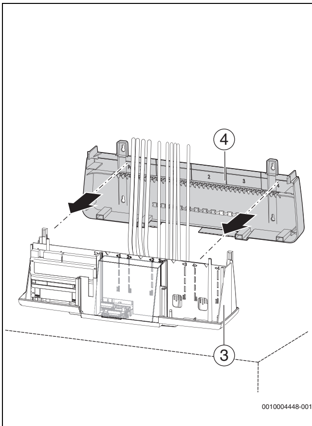
Sl.35 Pričvršćivanje stražnje stranice na donjem dijelu kućišta
