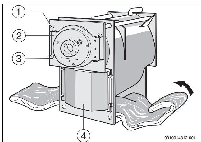
Sl.9 Toplinsku izolaciju provući ispod kotla
