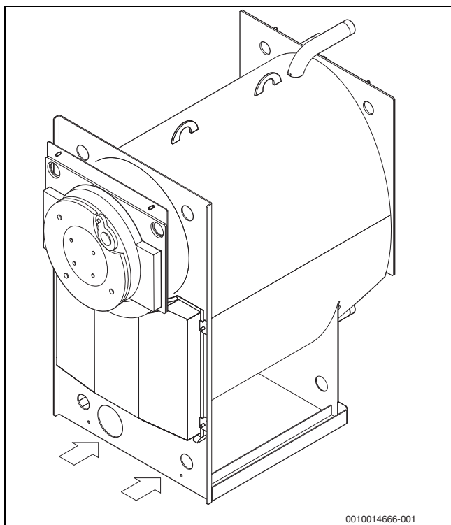
Sl.5 Transport kotla na viličaru
