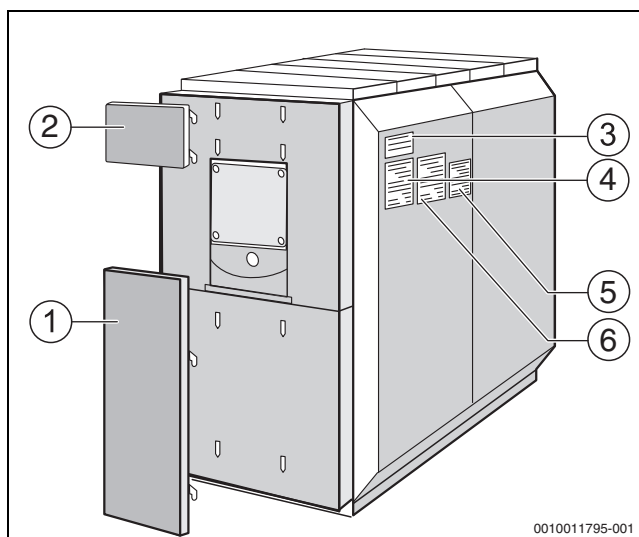
Sl.24 Pričvršćenje tipske pločice
