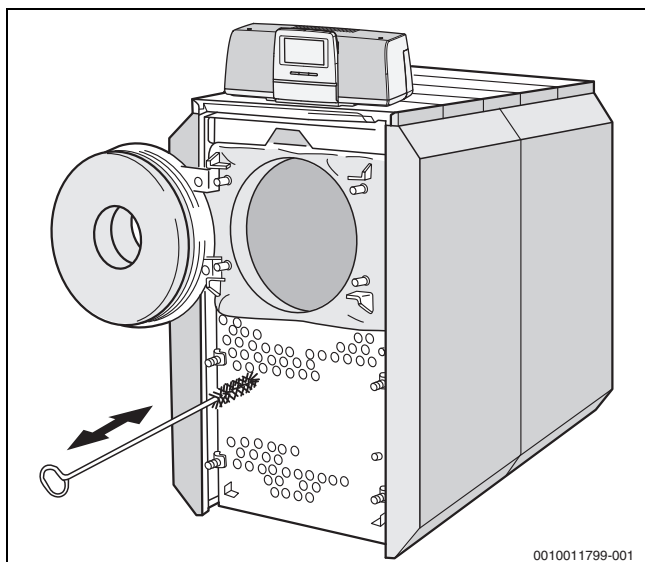
Sl.41 Čišćenje kotla četkom za čišćenje
