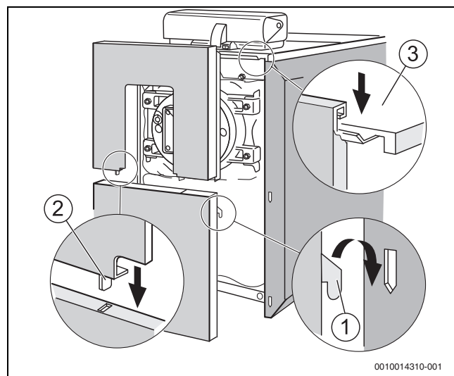
Sl.22 Pričvršćenje gornje i donje prednje stijenke
