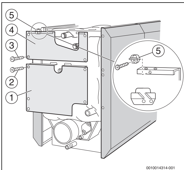
Sl.20 Pričvrstiti 2-dijelnu stražnju stranicu
