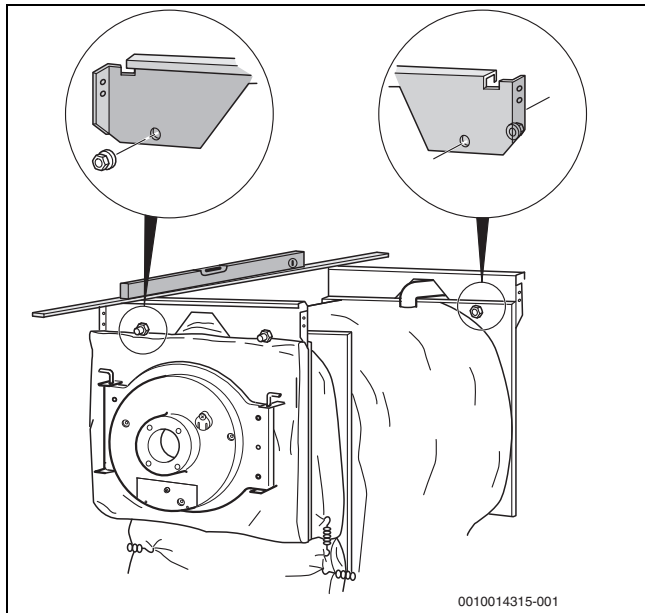
Sl.16 Prednju i stražnju traverzu umetnuti i pričvrstiti vijčano
