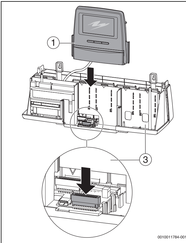
Sl.37 Umetanje upravljačke jedinice na donji dio kućišta
