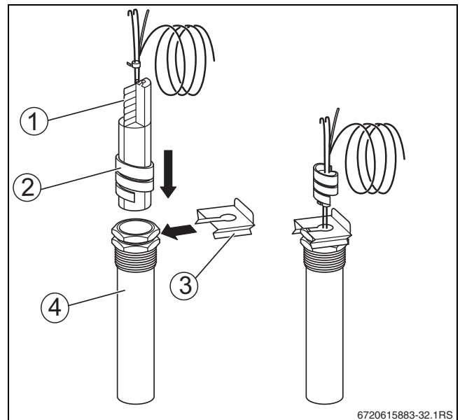
Sl.26 Umetanje plastične spirale u uronsku čahuru
