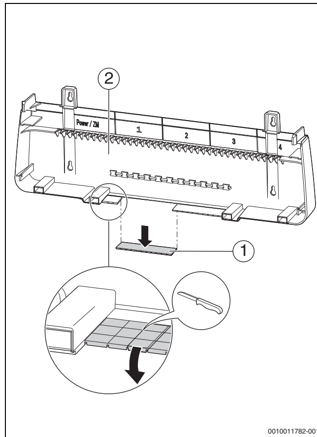
Sl.34 Priprema kabelske uvodnice
