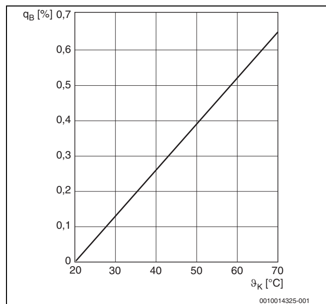
Sl. 46 Gubitak u pripravnom stanju ovisno o srednjoj temperaturi vode kotla
