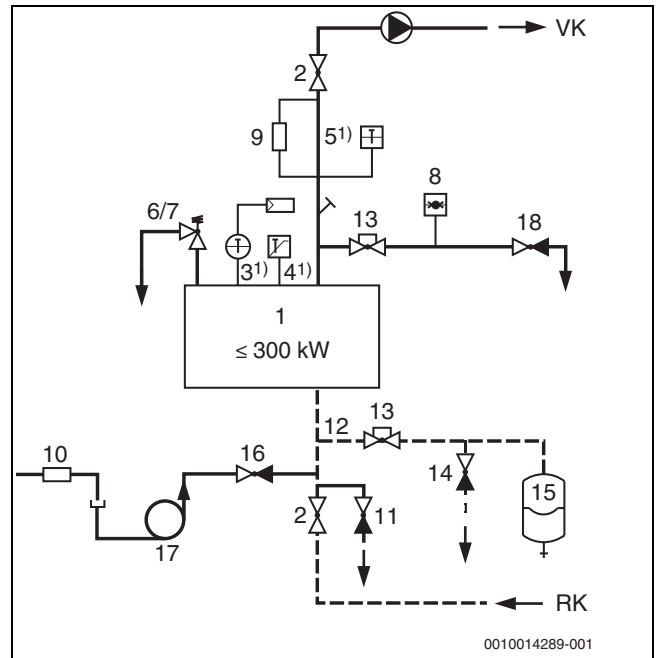
Sl.44 Sigurnosno-tehnička oprema prema EN 12828:2012 za kotao ≤ 300 kW sa sigurnosnim graničnikom temperature (STB) ≤ 110 °C
