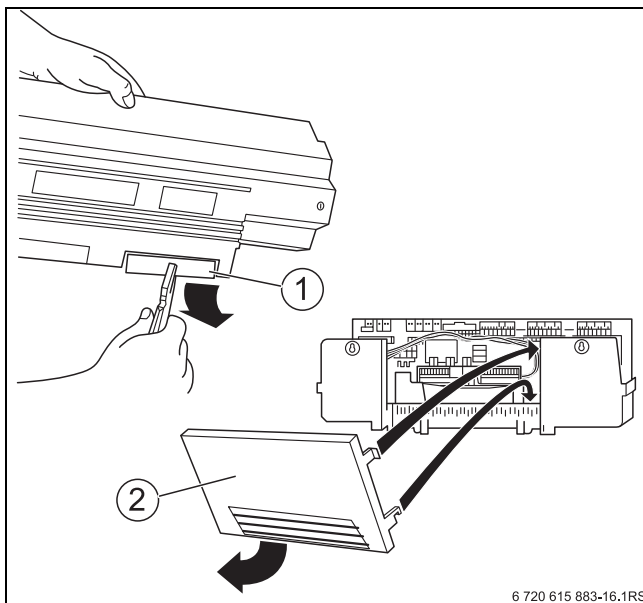
Sl.28 Priprema kabelaške ulaznice
