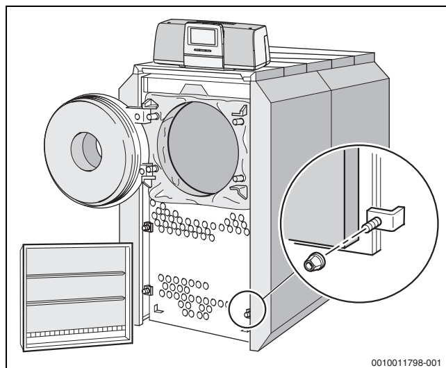
Sl.40 Skinuti poklopac za skretanje te otvoriti vratašca ložišta
