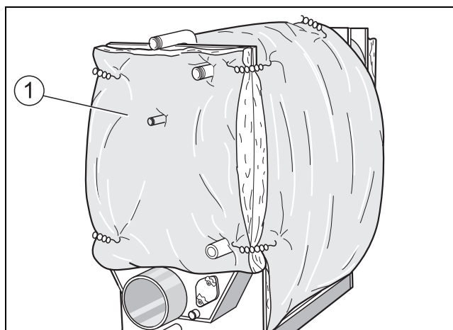
Sl.11 Stavljanje i pričvršćivanje toplinske izolacije stražnje stranice
