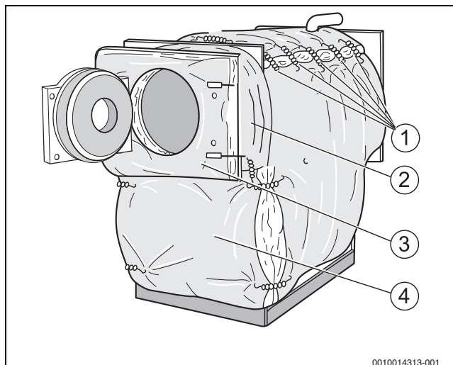
Sl.10 Stavljanje i pričvršćivanje toplinske zaštite
