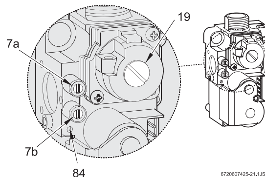
Sl. 5 Plinska armatura
