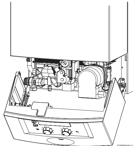
Sl. 4 Servisni položaj za podešenja plina
